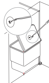
Podwieszenie pokrywy Suspension cover / Подвеска крышки
