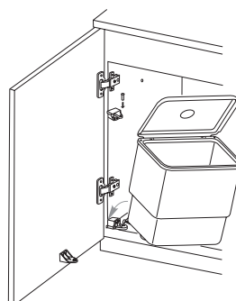
Sposób montażu Instruction of installation / Способ монтажа
