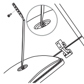
Podwieszenie pokrywy Suspension cover / Подвеска крышки
