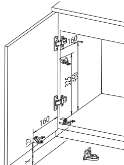
Wymiary montażowe Mounting dimensions / Монтажные размеры
